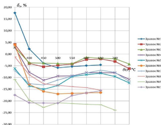
Рисунок 2 – Залежність відхилення \delta_{t,cul} від критичної температури сталі \theta_{cr} для реактивного вогнезахисного матеріалу
