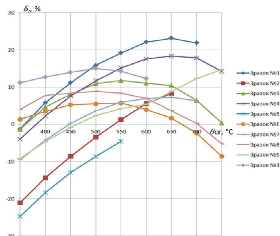
Рисунок 3 – Залежність відхилення \delta_{t,cul} від критичної температури сталі \theta_{cr} для пасивного вогнезахисного матеріалу
