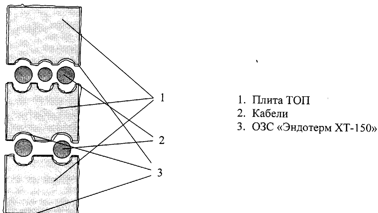
Рисунок 2. Схематичное изображение частей кабельной проходки перед началом сборки
